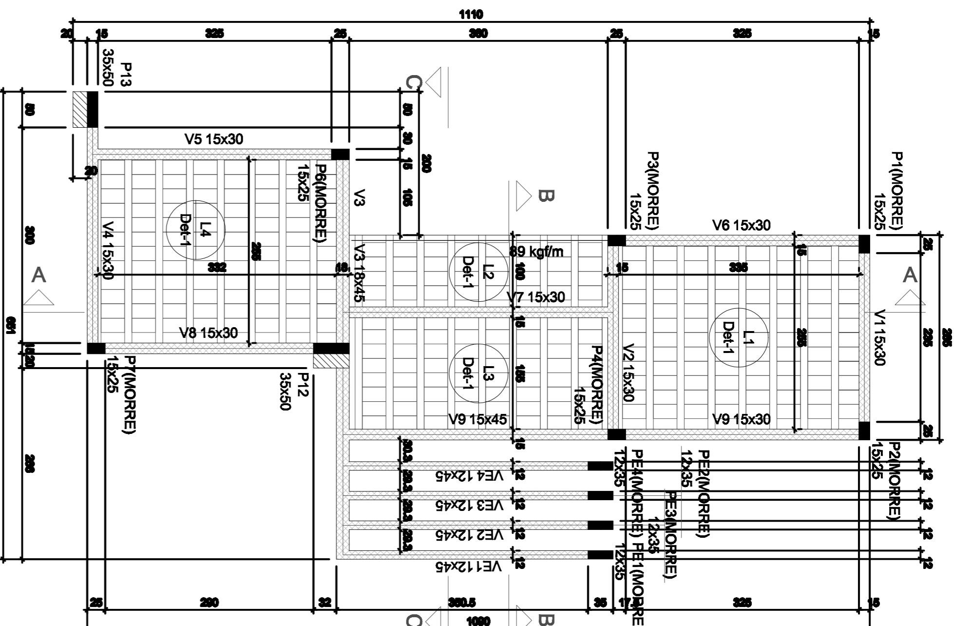
Forma do pav. Vigas de Coberta (Nível 382) escala 1:50
